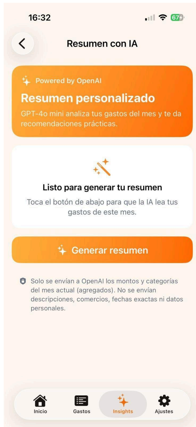
Figura 8. Pantalla del resumen con IA antes de generar. Incluimos un disclaimer explícito sobre los datos que se envían a OpenAI, reforzando el principio de IA centrada en el humano.
