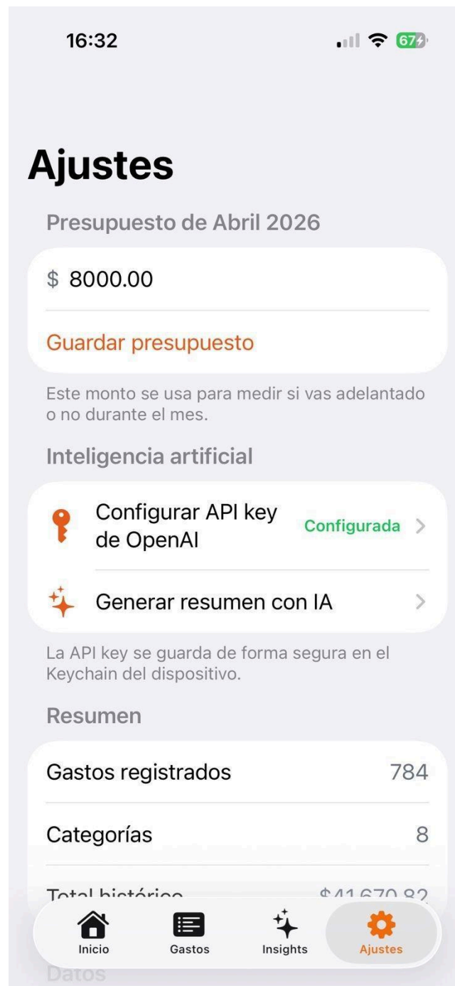
Figura 12. Pantalla de Ajustes con presupuesto editable, sección de Inteligencia artificial y resumen estadístico. La indicación "Configurada" en verde confirma que la API key fue guardada en el Keychain.
